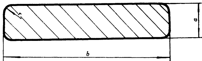
窄边 a 宽边 b 圆角半径 r
