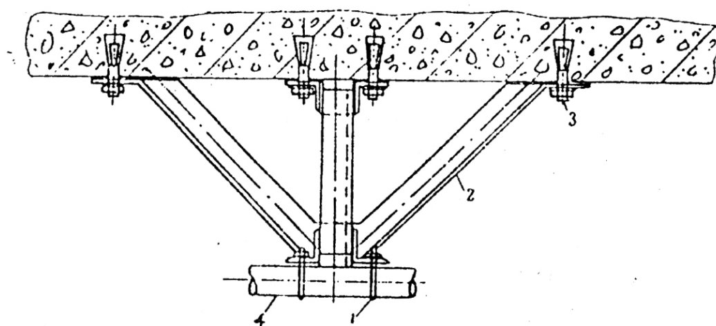
固定支架
