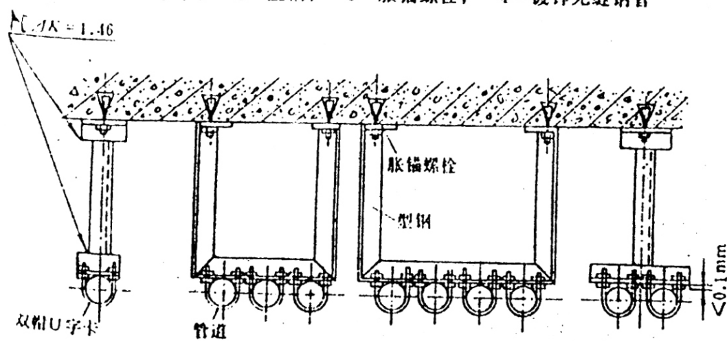
活动支架
