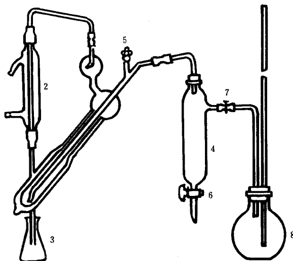
凯氏微量蒸馏装置图
